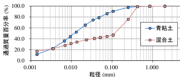
図-1 各試料の粒度分布
