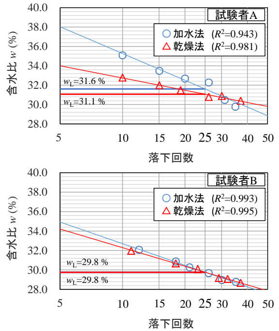
図-3 混合土における各試験者の液性限界試験結果
