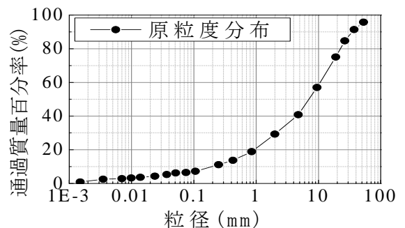
図1 試験試料の粒度分布
